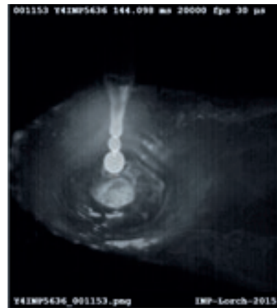
la goutte primaire est dirigée dans le bain de fusion et les gouttes secondaires se dissolvent.
