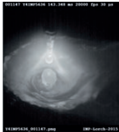
la goutte primaire s'est dissoute et les gouttes secondaires se forment.
