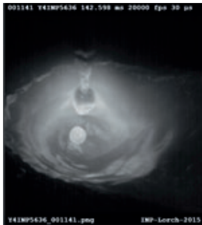
la goutte primaire se forme à l'extrémité du cordon.
