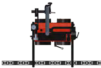
Schweißen: Brennerseite gegenüberliegend zur Flex-Führung
