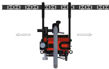
Schweißen: Brennerseite hin zur Flex-Führung
