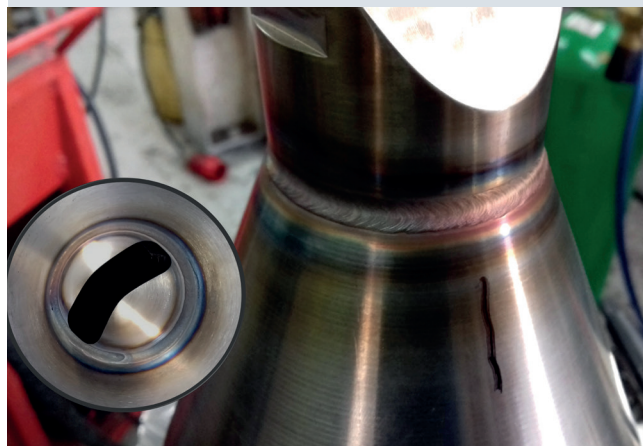
Ventil s rotačním svarem
