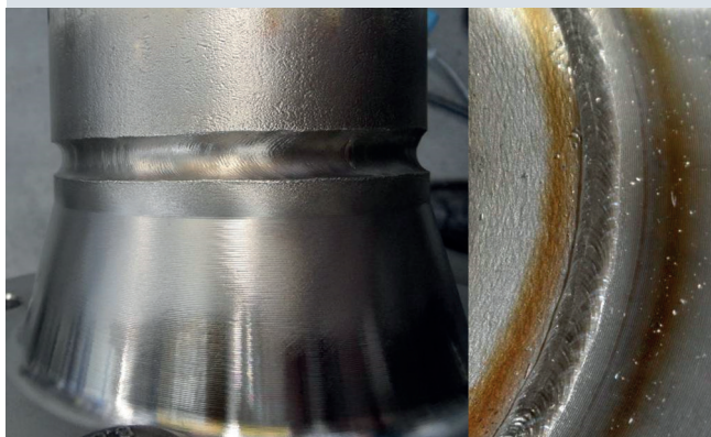
Kořen příruby
